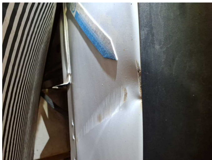
Beschädigung 15: Karosserie: C-Säule rechts - Delle / Lackschaden - instandsetzen und lackieren
