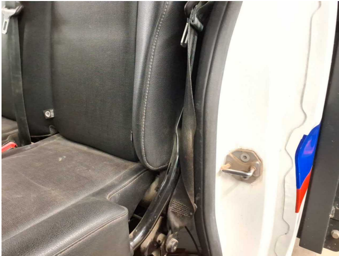
Beschädigung 7: Gurtsystem hinten: Sicherheitsgurt hinten rechts (+ hinten links) - Fehlstellung - instandsetzen
