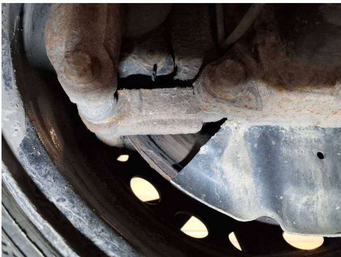
Beschädigung 17: Bremsanlage: Bremsscheiben und Beläge hinten (Tragbild) - Korrosion - erneuern
