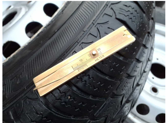
Beschädigung 14: 2.Radsatz: 2 Reifen - verschlissen - erneuern
